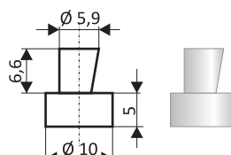
Razník Typ B
