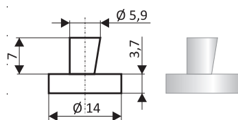
Razník Typ A - nejpoužívanější
