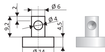
Razník Typ C
